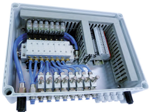
Vezérlődoboz elektromos vezérlésű szelepekkel etetők működtetéséhez
